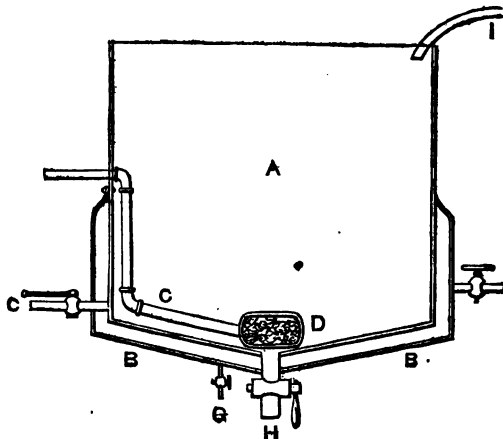
Air Agitator.
